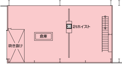
2階平面図
